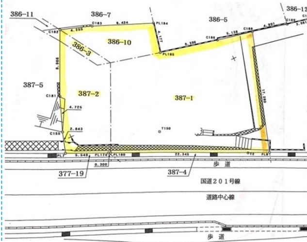
地積測量図
