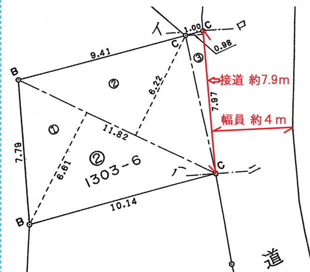
測量図
