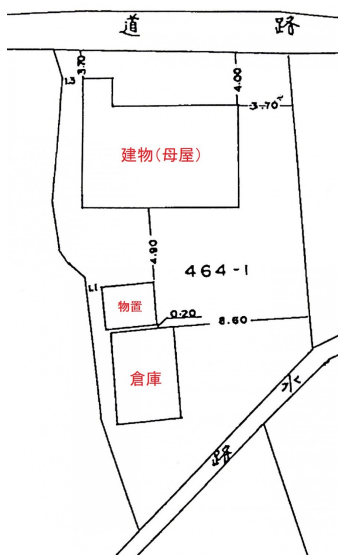
配置図
